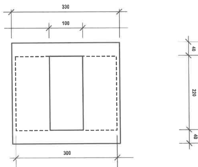
Hatos sírbolt járda méretei
