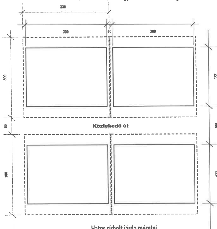
Hatos sírbolt méretei és egymástól való távolsága
